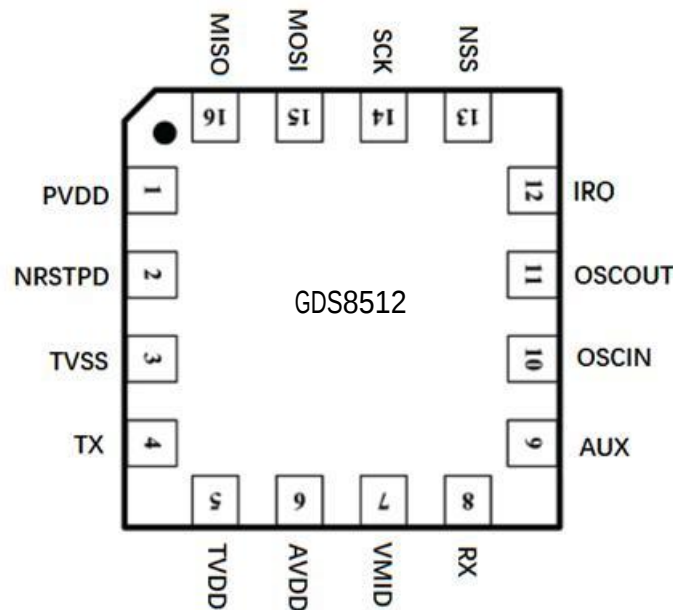
图 1 QFN16 封装管脚图
